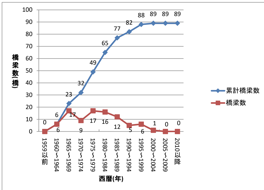
図-1 累計橋梁数の推移
